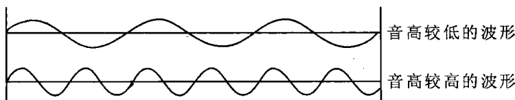
图 1-2 音高:对应于频率高低
