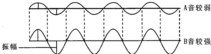
图 1-3 音强对应于振幅的大小
