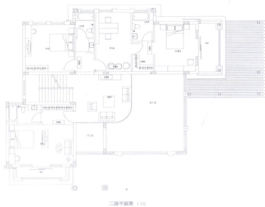
二层平面图 1:50
