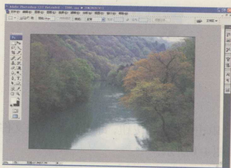
图 3-2 素材图像
