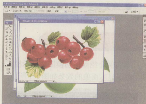
图 9-3 层叠效果
