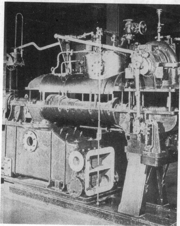
1901年的汽轮发电机
