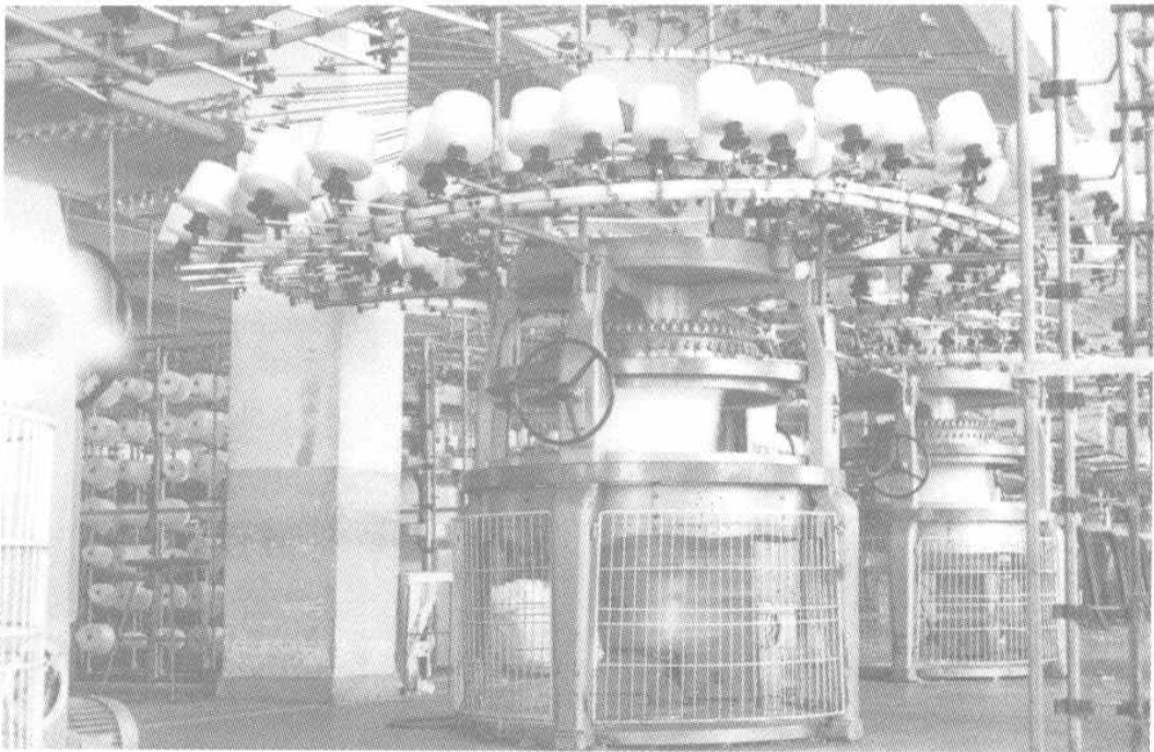
大连针织厂 1984 年从日本、美国等国家引进大园机 44 台
