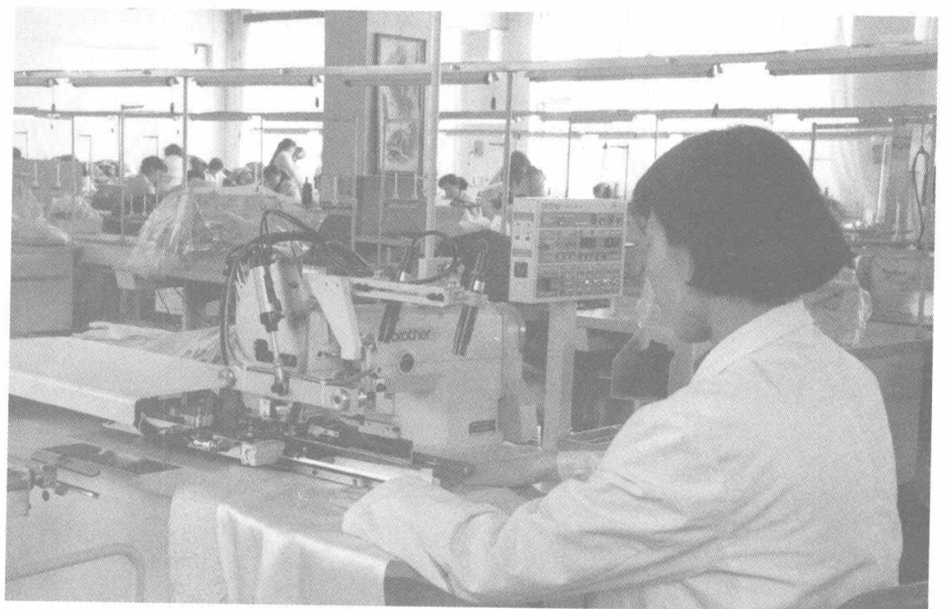
大连第三呢绒服装厂引进世界最先进的日本电脑控制自动开袋机
