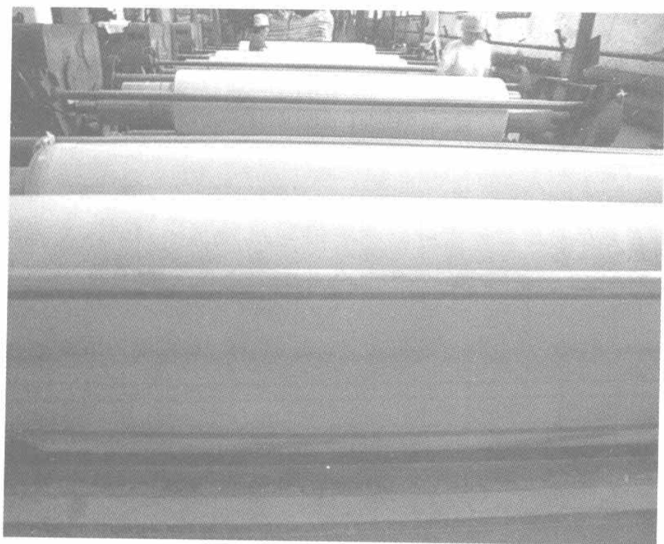
大连提花织物厂购置国产先进的染整加工生产线,图为漂染车间
