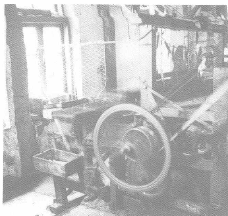
合营前使用的皮带传动“木架子机”,也称“跳舞机”、“扭秧歌机”
