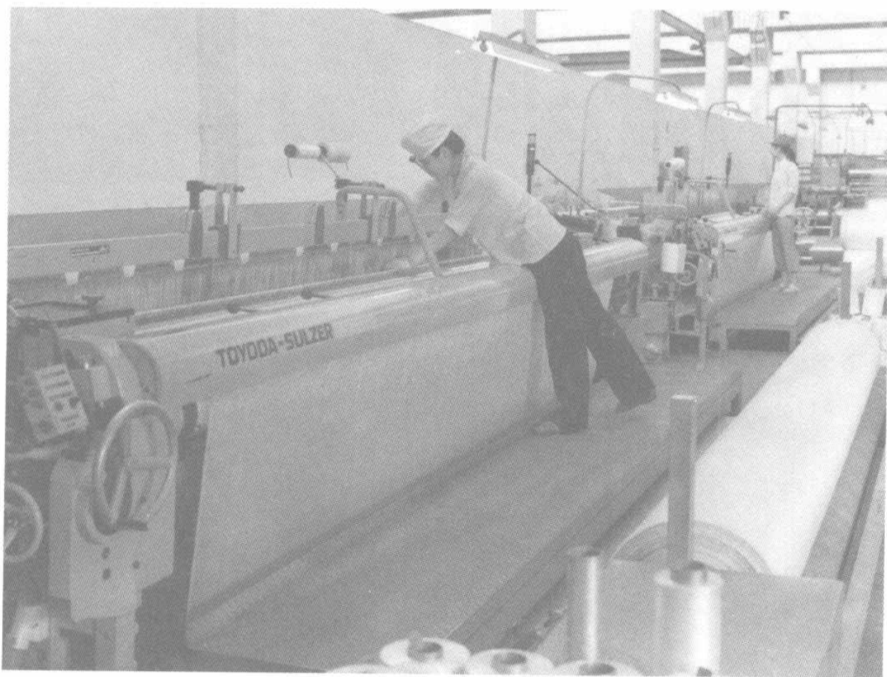
大连麻纺织厂引进用于生产地毯底布的片梭织机
