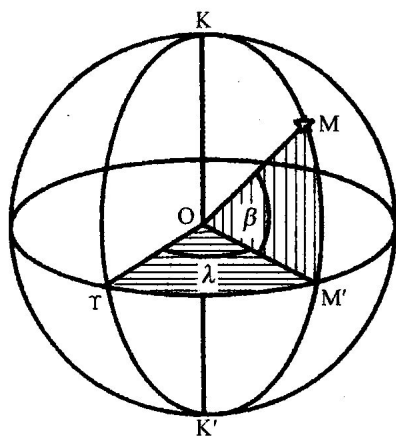
图 1-8 黄道坐标系
