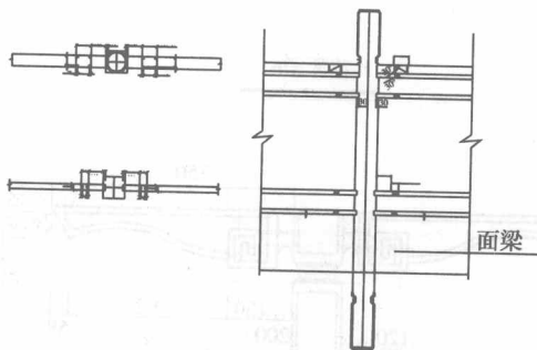
横枋混凝土柱连接大样
