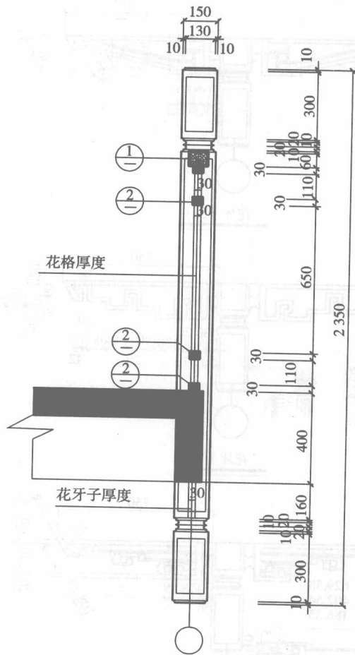
A—A剖面图
