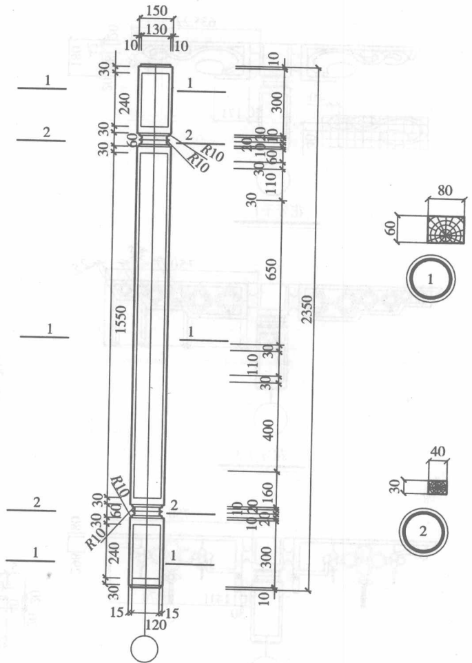
立柱大样图
