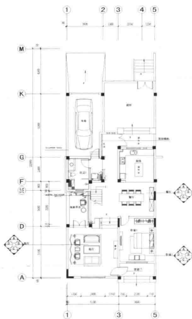
一层平面布置图
