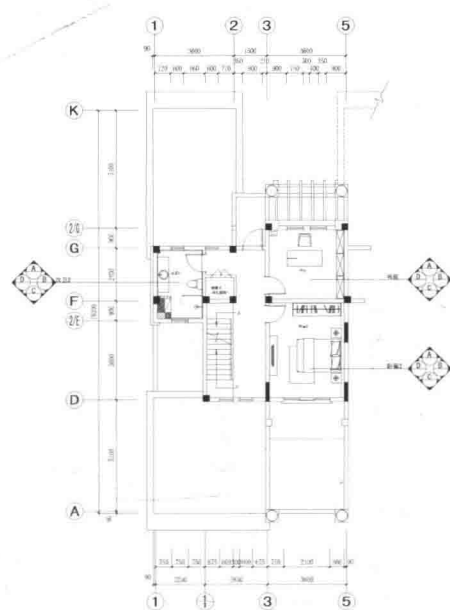
二层平面布置图
