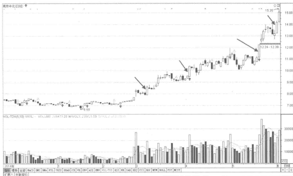
图 1-5 阳线实体大小比较示意图
