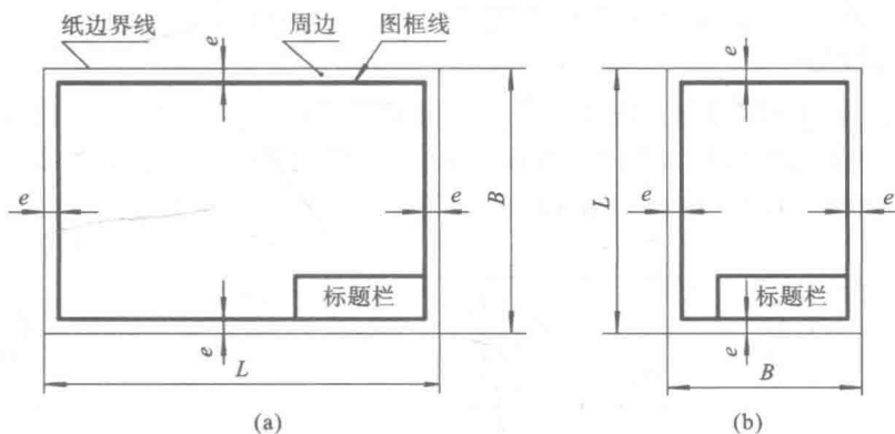
图 1-3 不需要装订图样的图框格式
