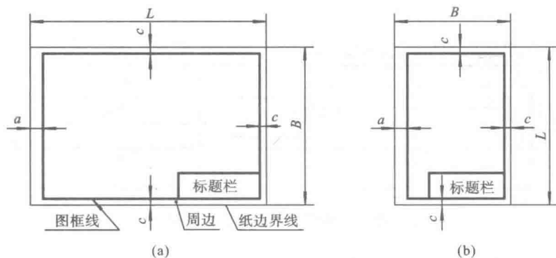
图 1-2 需要装订图样的图框格式
