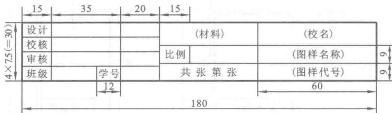
图 1-5 制图作业用简化标题栏格式
