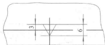
图 1-7 方向符号的画法
