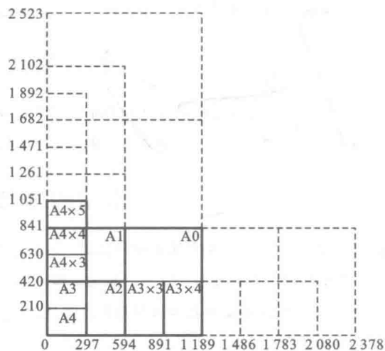
图 1-1 基本幅面与加长图纸幅面
