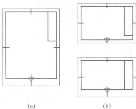
图 1-6 标题栏的方向
