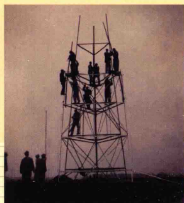
高钢觇标建造中
