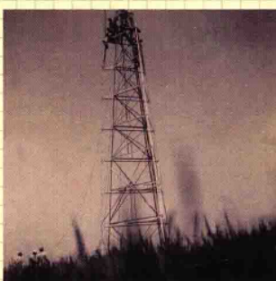
高钢觇标建造过半
