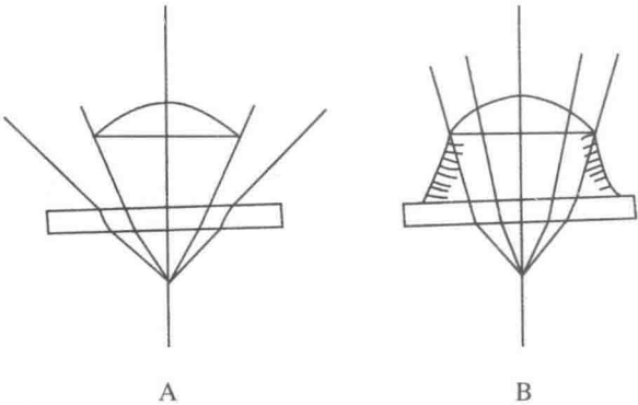
图 1-1 油镜头的原理
