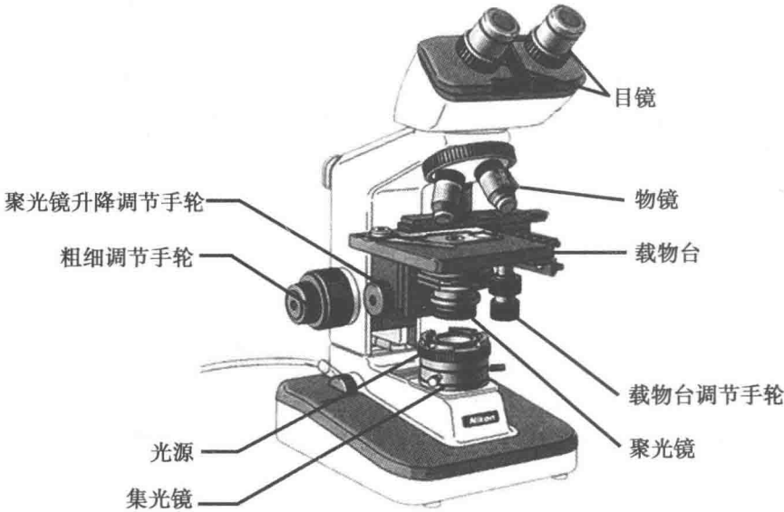
图 1-2 显微镜的结构
