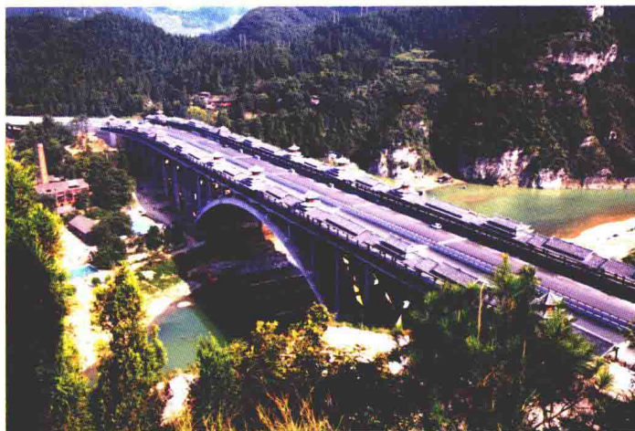
建成后的清水江风雨桥
