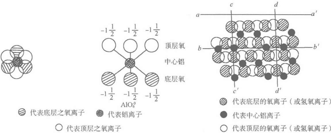
图 2 - 2 铝氧八面体和铝氧片的构造示意图
