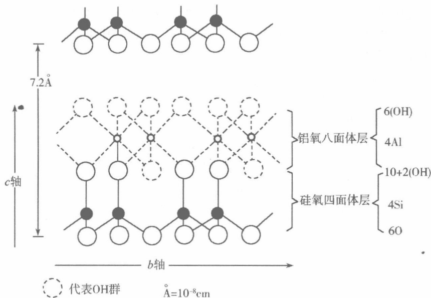
图 2 - 3 1 : 1 型层状硅酸盐矿物高岭石的结构示意图
