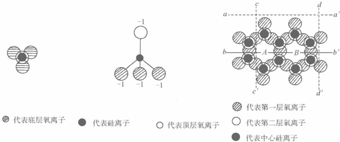
图 2-1 硅氧四面体和硅氧片的构造示意图
