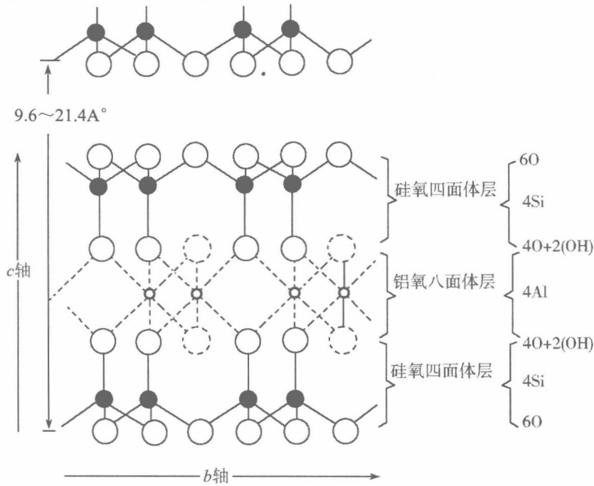
图 2 - 4 2 : 1 型层状硅酸盐矿物蒙脱石的结构示意图
