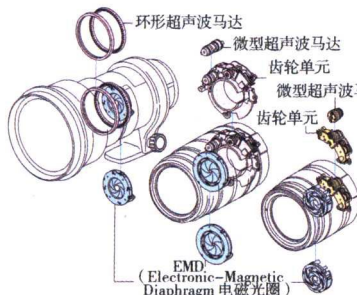
EF 镜头所采用的 3 种超声波马达·USM
