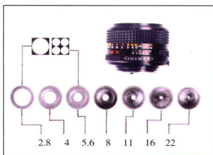
2-3 光圈示意图
