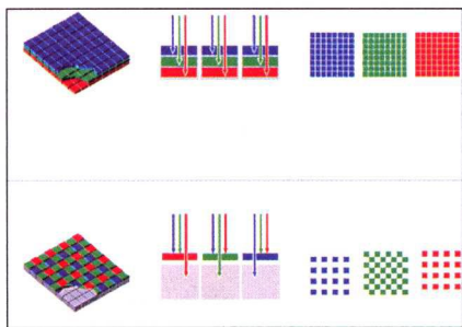
1-13 Foveon×3传感器与普通传感器比较
