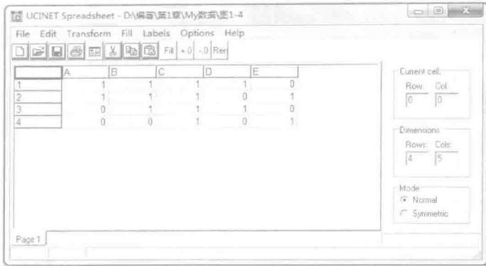
图 1-5 (a) 用“数据编辑器”输入初始发生阵
