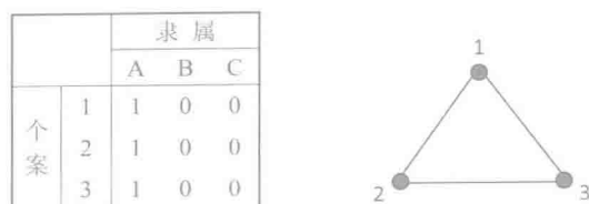
图 1-2 一个简单的关系矩阵及其社群图
