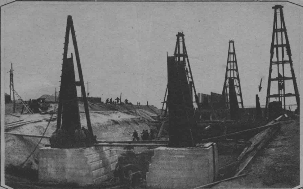
橋墩全景
