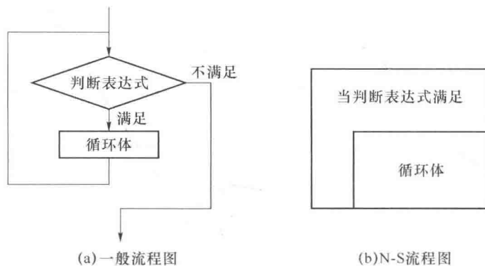
图 1-4 当型循环
