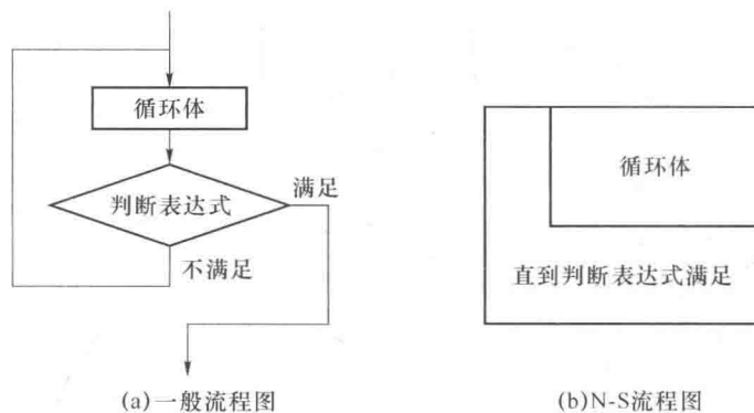
图 1-5 直到型循环
