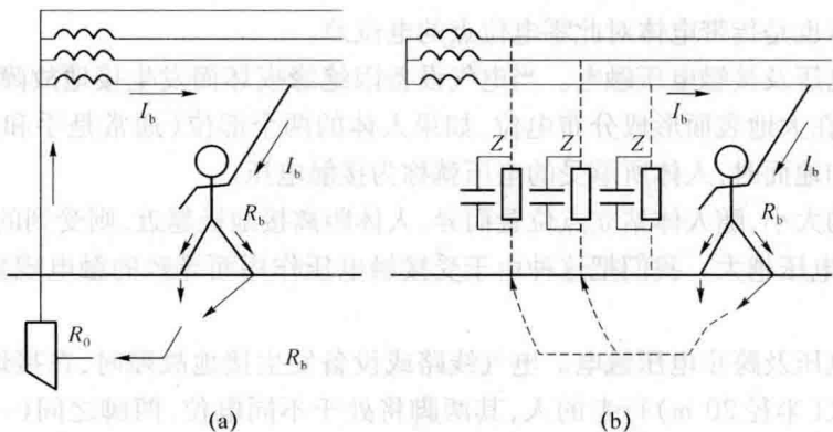
图1-1-1 单相触电示意
