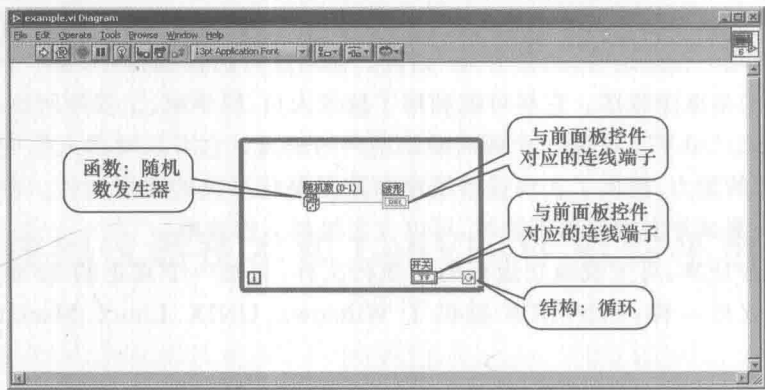
图 2-3 随机信号发生器的框图程序
