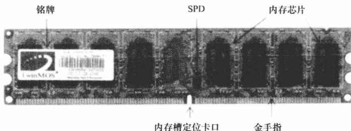
图 1-3 内存条
