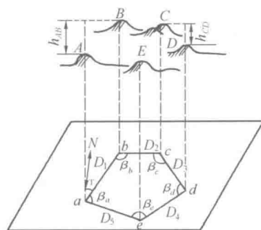
图 1-5 地面点的空间位置
