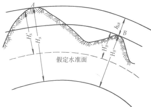
图 1-3 大地水准面
