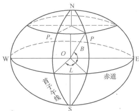
图 1-2 大地坐标
