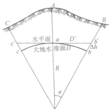
图 1-4 水平面代替水准面对距离和高程的影响
