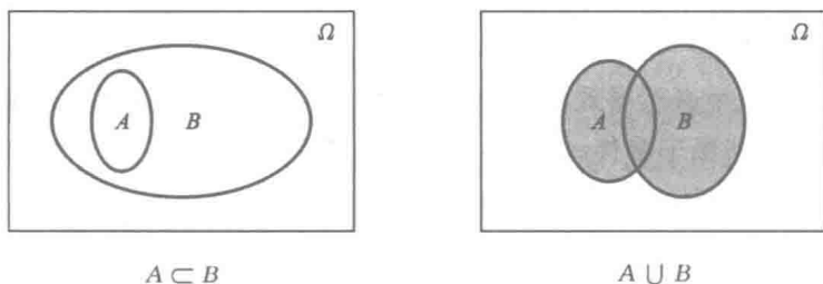
图 1-1 事件关系与运算关系韦氏图
