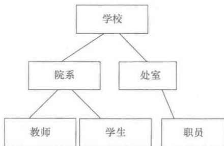
图 1-6 层次模型
