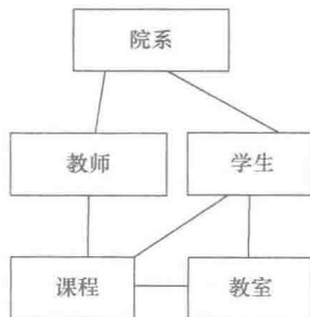
图 1-7 网状模型
