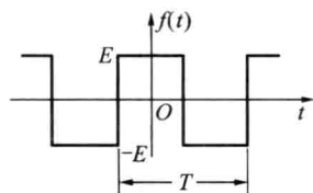
图 1-6 周期性方波信号
