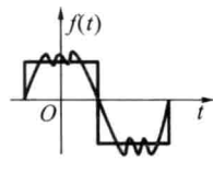
(c) 基波和3次谐波、5次谐波合成
