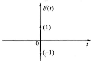
图 1-13 冲激偶 \delta'(t)
