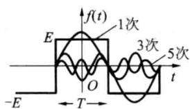
(a) 方波的分解
