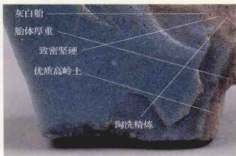
图5 厚胎钧瓷标本 宋代。
