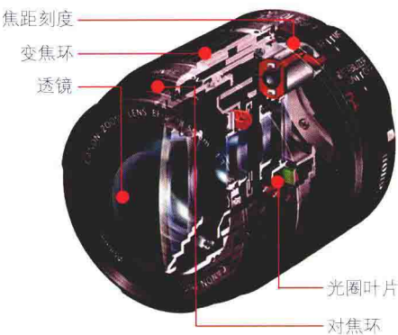
镜头结构示意图
