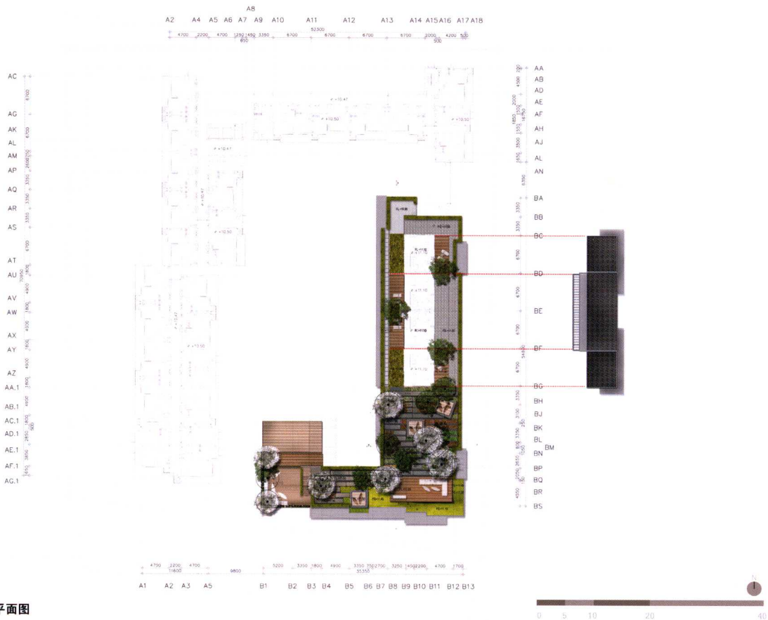
屋顶植物平面图
