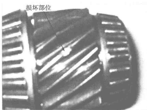
图 1-4 齿轮副损坏
