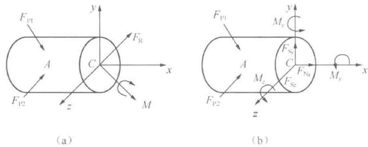
图 1-17 内力分量
