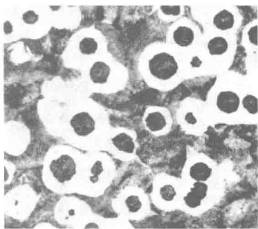
图 1-9 球墨铸铁的显微组织
