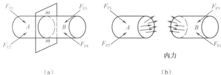
图 1-13 截面法
