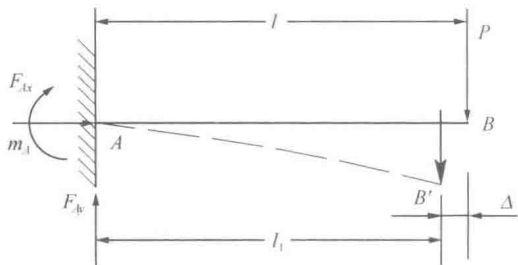
图 1-12 小变形假设
