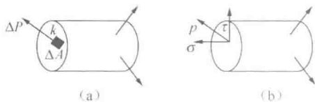
图 1-15 应力表示
