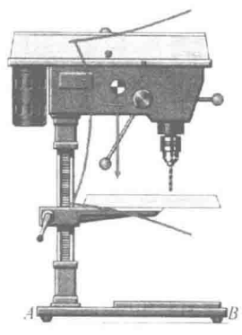
图 1-6 钻床立柱刚度不足示例
