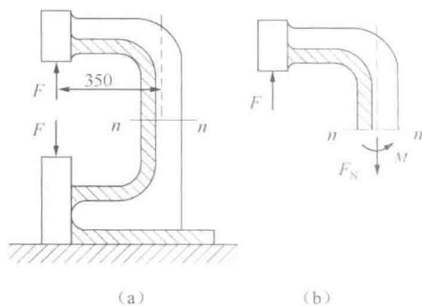
图 1-14 例 1-1 图
