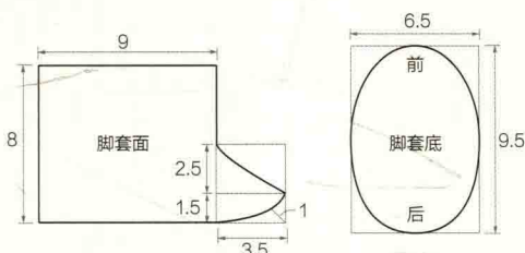
裁剪图
