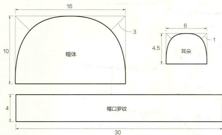
裁剪图
