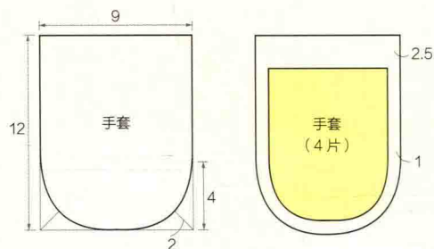
裁剪图
