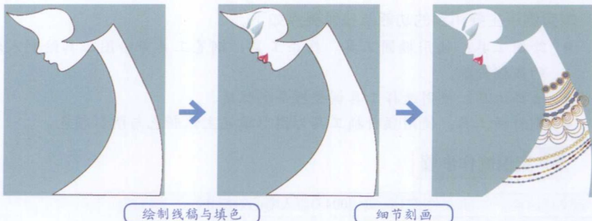
图1-18 效果展示
