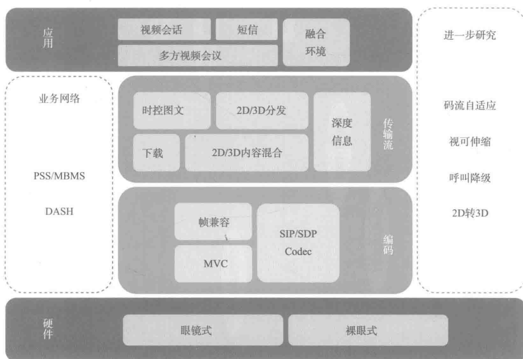
（关键技术二）图5-2-1 3GPP Mobile 3D协议架构
