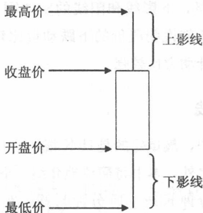
图 1-2 阳线
