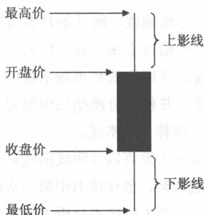
图1-1 阴线
