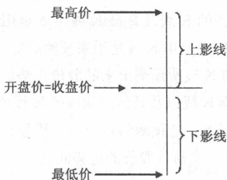
图 1-3 平线
