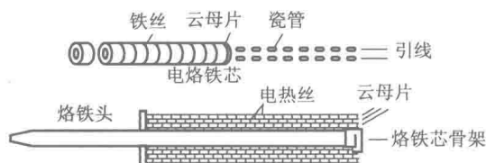
图 1-2 烙铁芯结构
