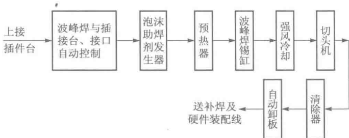
图1-6 波峰焊工艺流程
