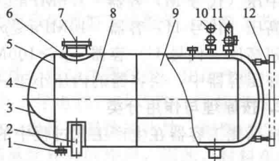
图 1-1 化工容器的基本结构
