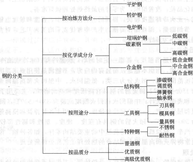
图 1-3 钢的分类
