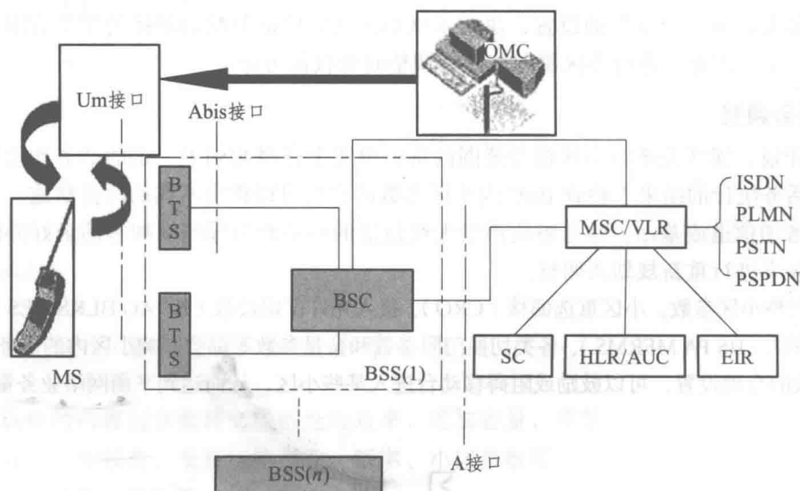
图 2.1 GSM 系统的组成
