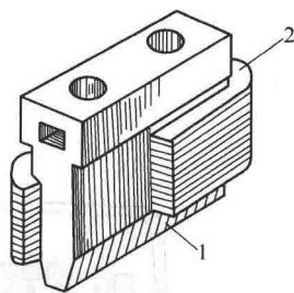
图 1-6 直流电机的换向极 1—换向极铁心 2—换向极绕组
