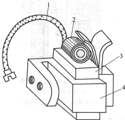
图 1-8 恒压刷握装置 1—铜丝辫 2—压紧弹簧 3—电刷 4—刷握
