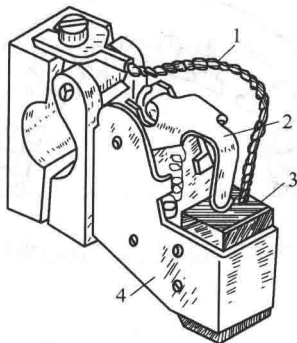
图 1-7 电刷与刷握装置 1—铜丝辫 2—压紧弹簧 3—电刷 4—刷盒
