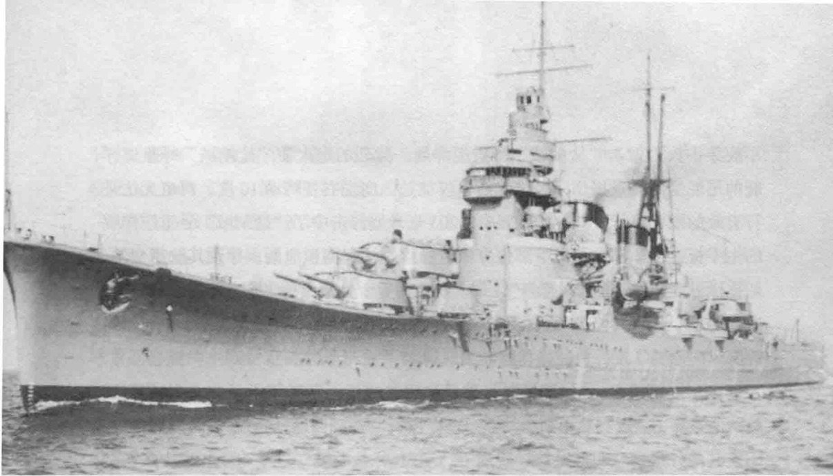
日本海军“妙高”级“那智”号重巡洋舰，以日本和歌山县的那智山命名。在科曼多尔群岛海战中，“那智”号重巡洋舰被击伤，11人阵亡、21人负伤。1944年11月5日，在菲律宾的马尼拉湾，它遭到美军航空母舰舰载机的空袭而沉没
