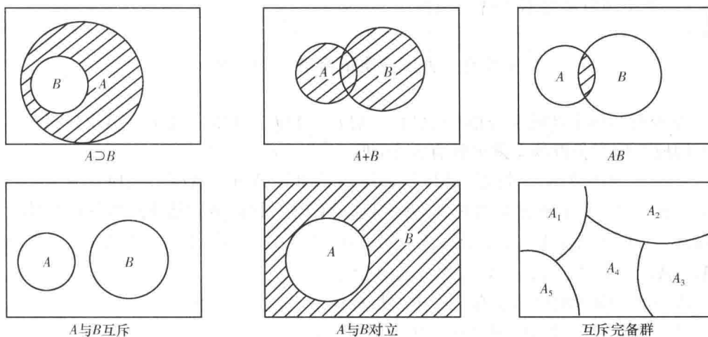
图 1-1 韦恩图
