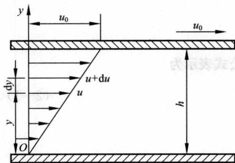
图 2-1 液体的黏性示意图
