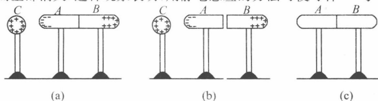
图 10.1.1 静电感应
