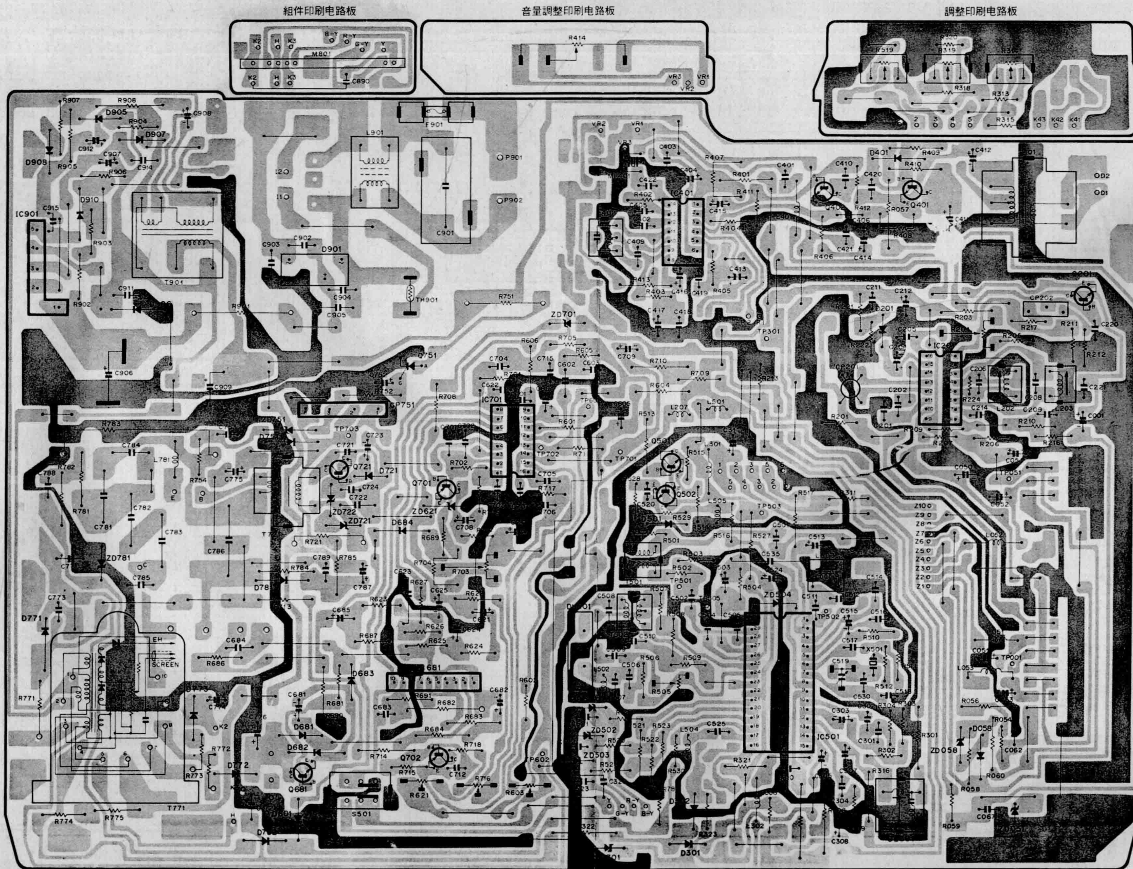
日立彩色 CRP451D 11"(CEP321D 18") (3) 印刷板图
