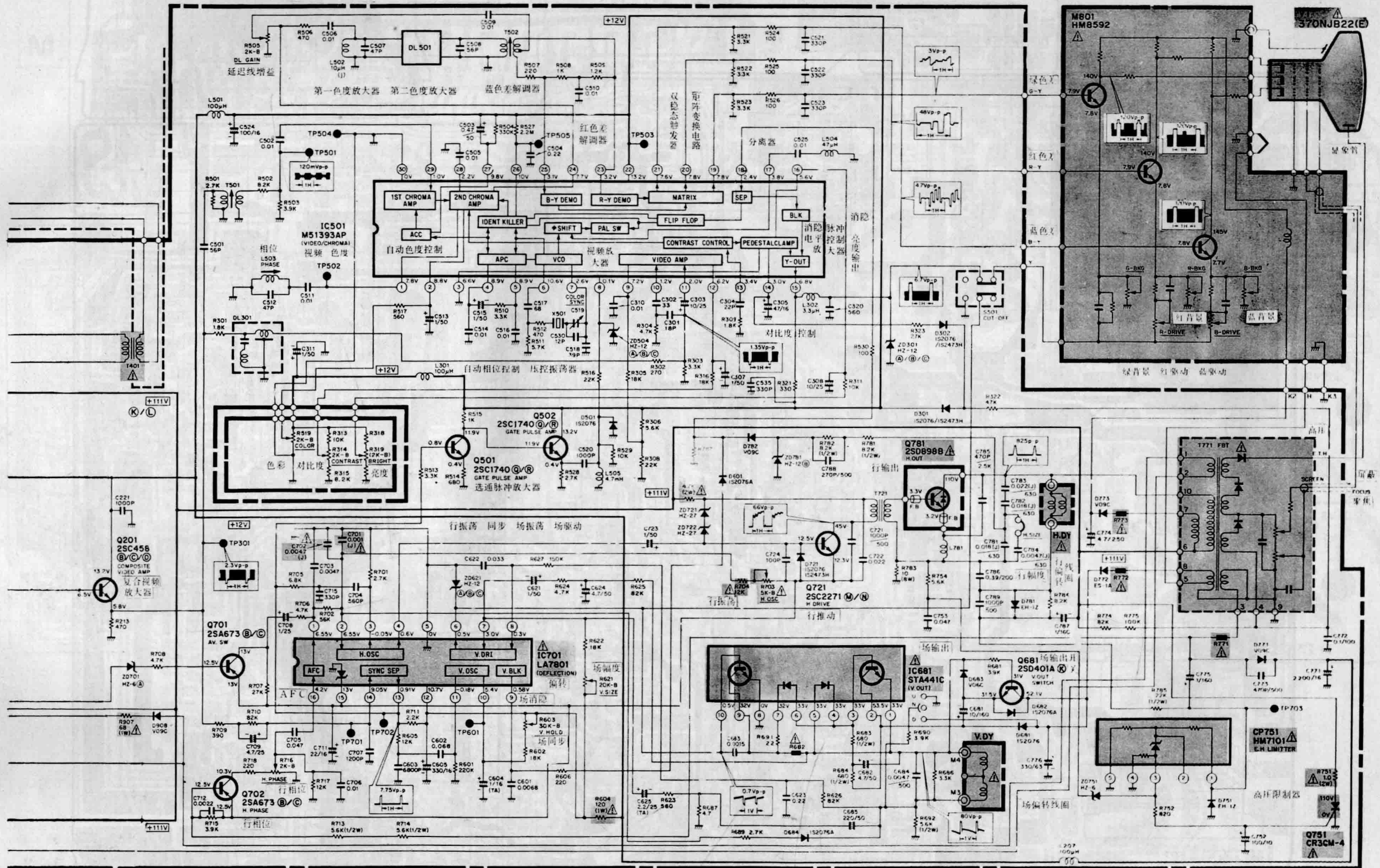
日立彩色 CRP 451D 11"(CEP321D 18") (2) 电路图
