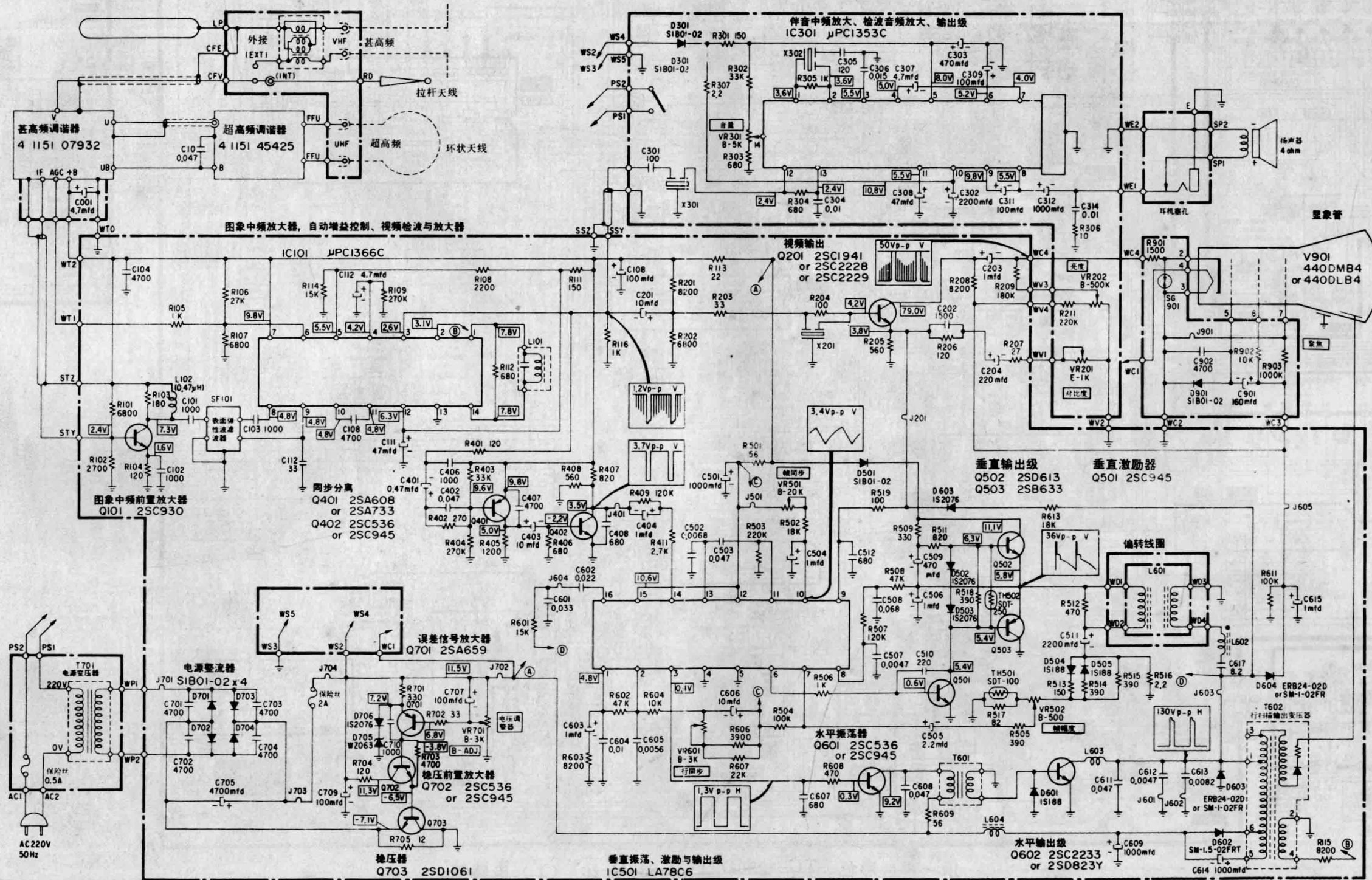
三洋黑白 17-T716U1 17" (1) 电路图
