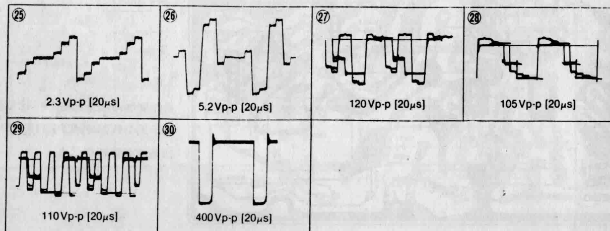
乐 声 彩色 TC—230D/TC—830D 20" (3) 调谐器及电压波形图
