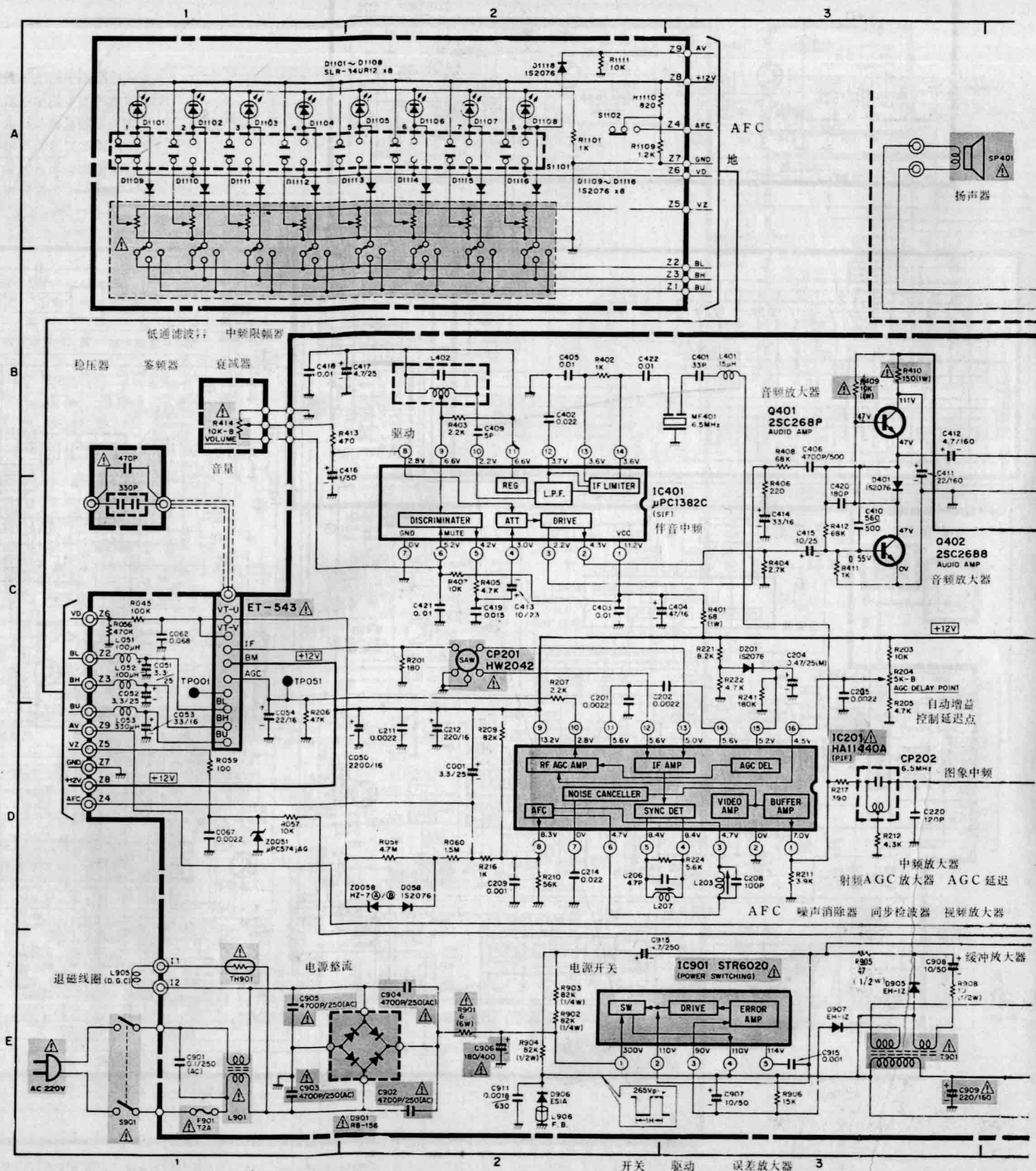
目 立 彩色 CRP 451D 14" (CEP321D18") (1) 电路图
