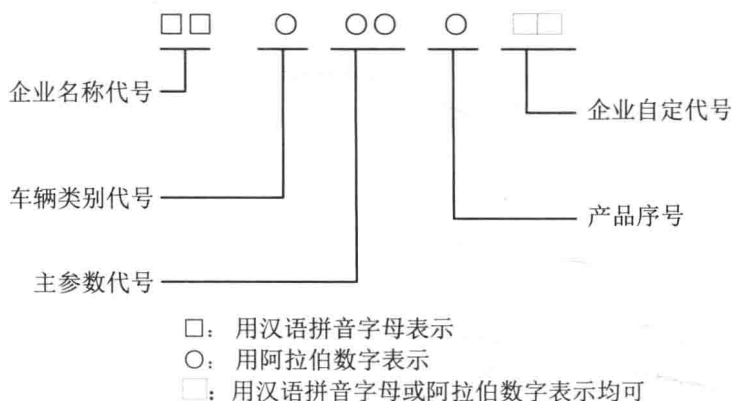
图 1-2 汽车型号组成示意图
