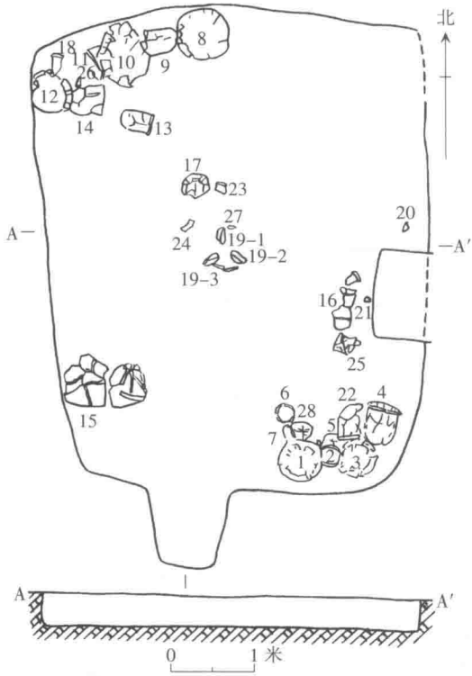
图四 章丘西河遗址 F58 平、剖面图
