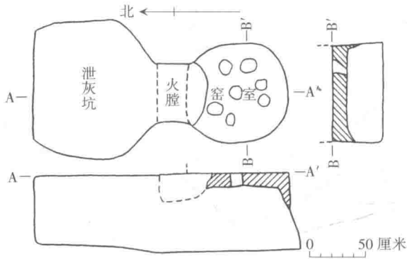
图五 临淄后李遗址 Y6 平、剖面图
