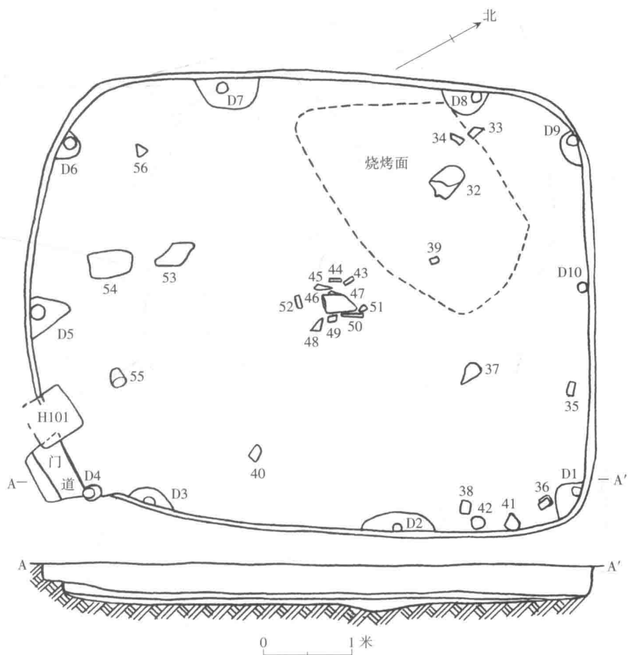
图三 章丘小荆山遗址 F11 平、剖面图
