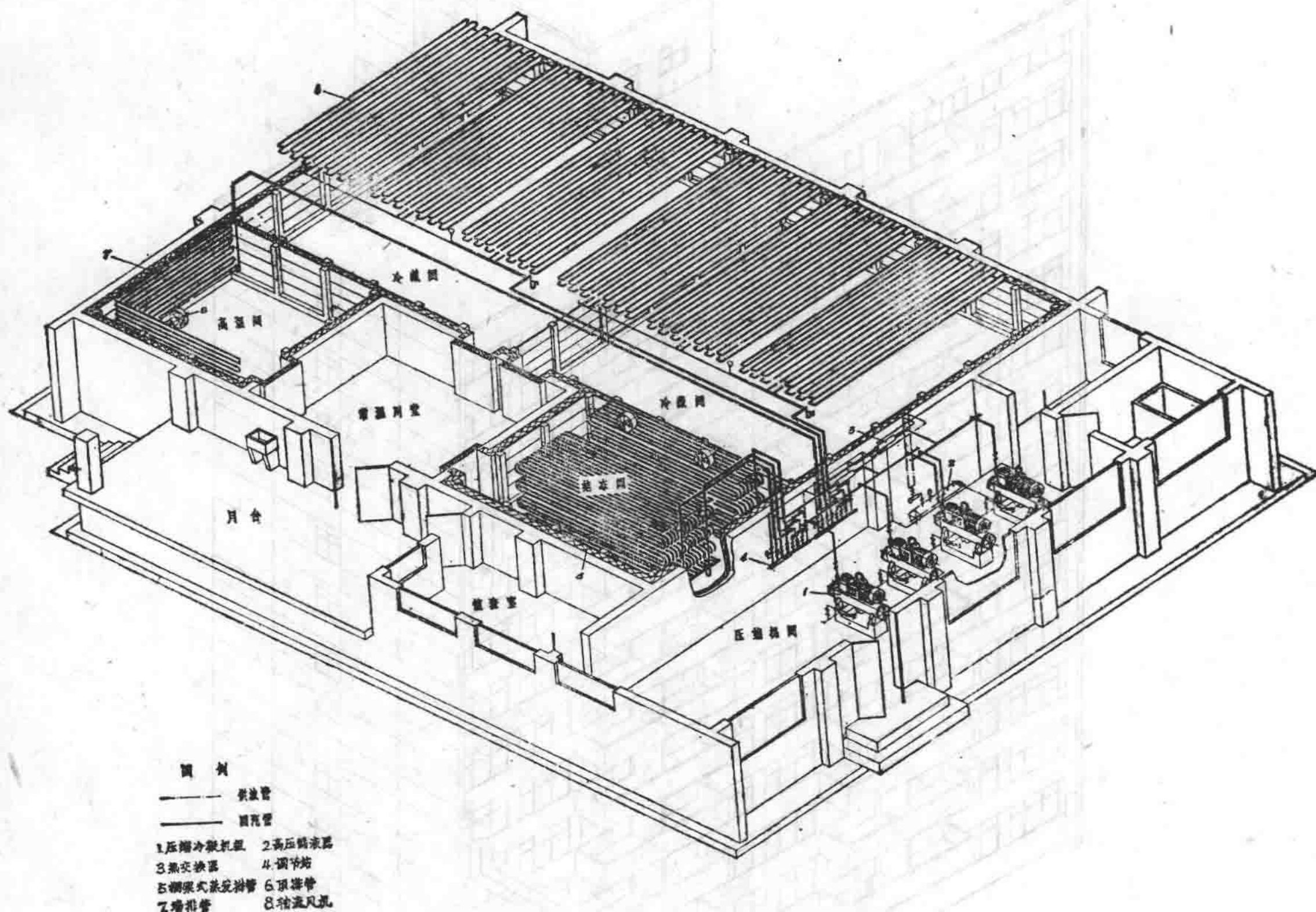
图 0.2 小型冷库制冷系统及其库房分布
