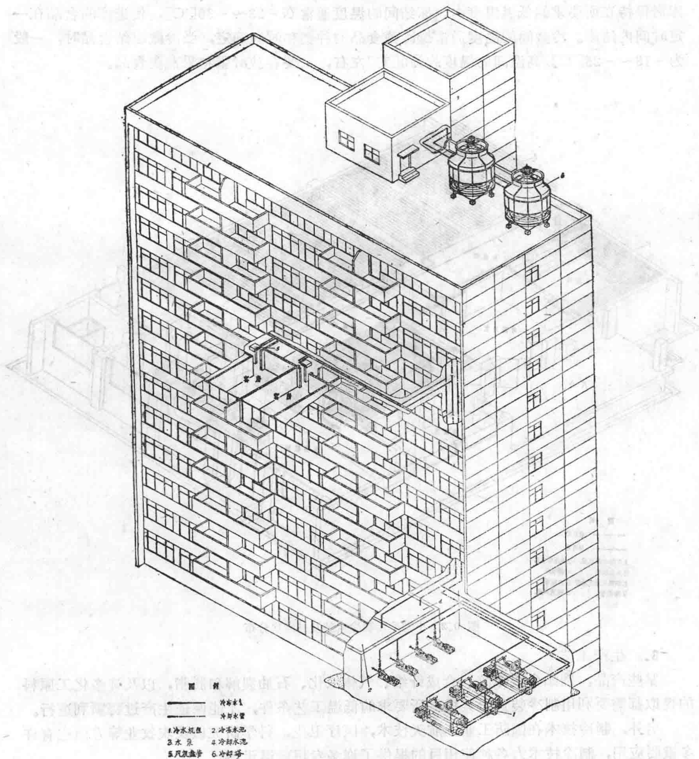
图 0.1 高层建筑制冷、空调系统图
