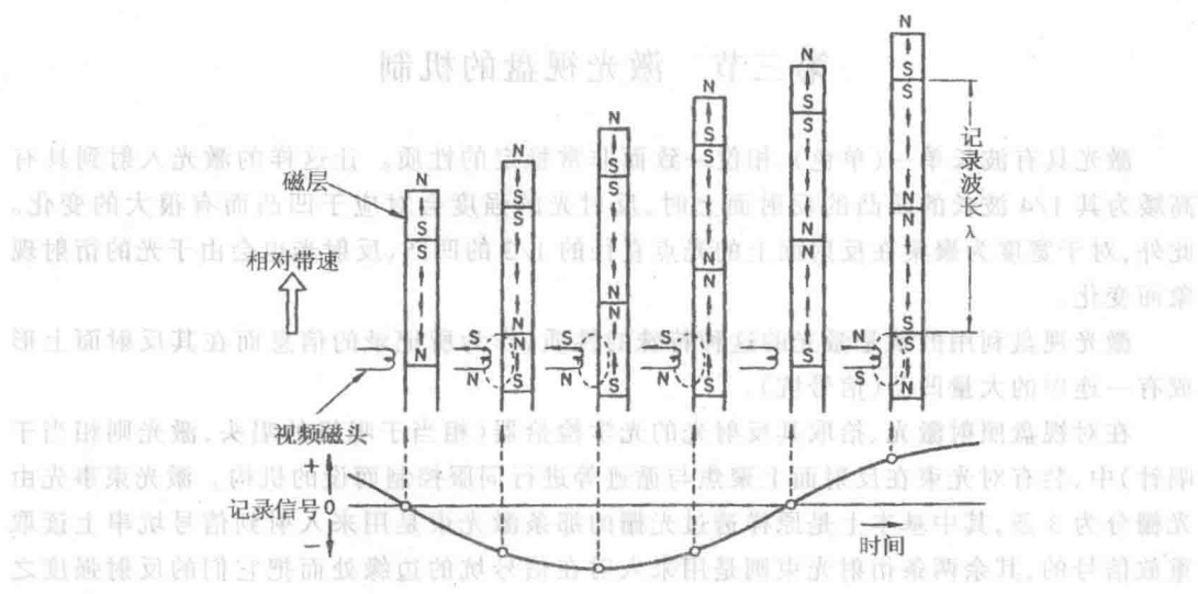
图 1-5 磁性记录的记录波长
