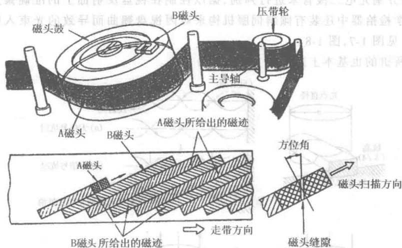
图 1-6 螺旋扫描方式
