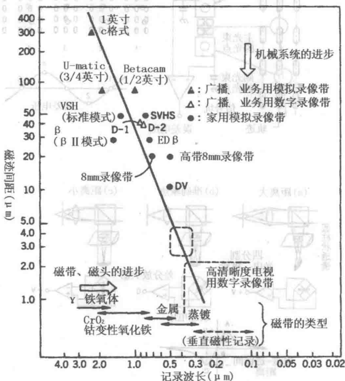
图 1-9 VTR 的高密度记录化的历史
