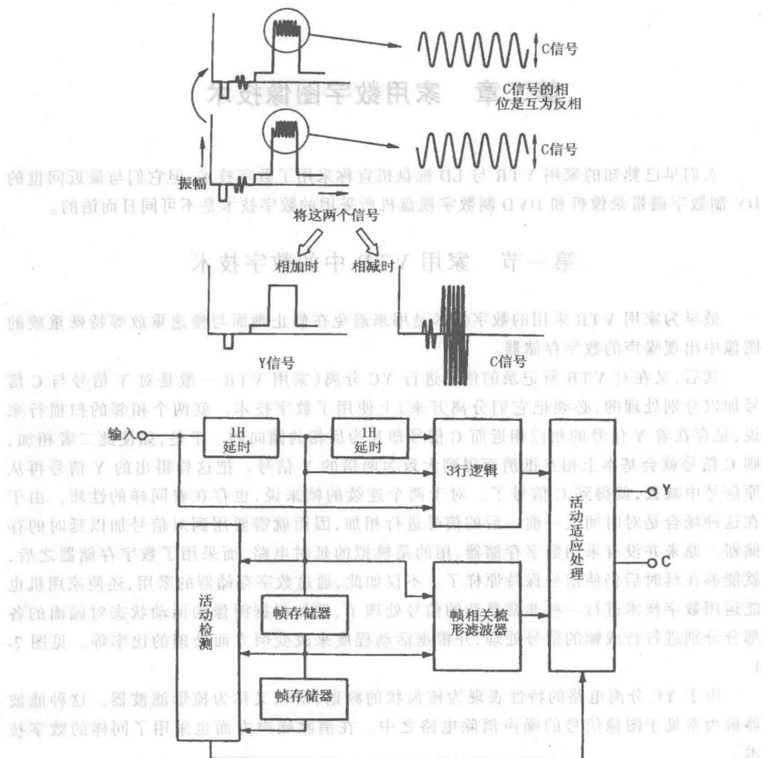
图 2-1 YC 分离(扫描行之间)的原理与三维数字 YC 分离
