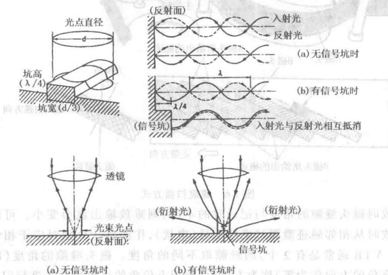
图 1-7 反射面上的信号坑所给出的反射光的变化
