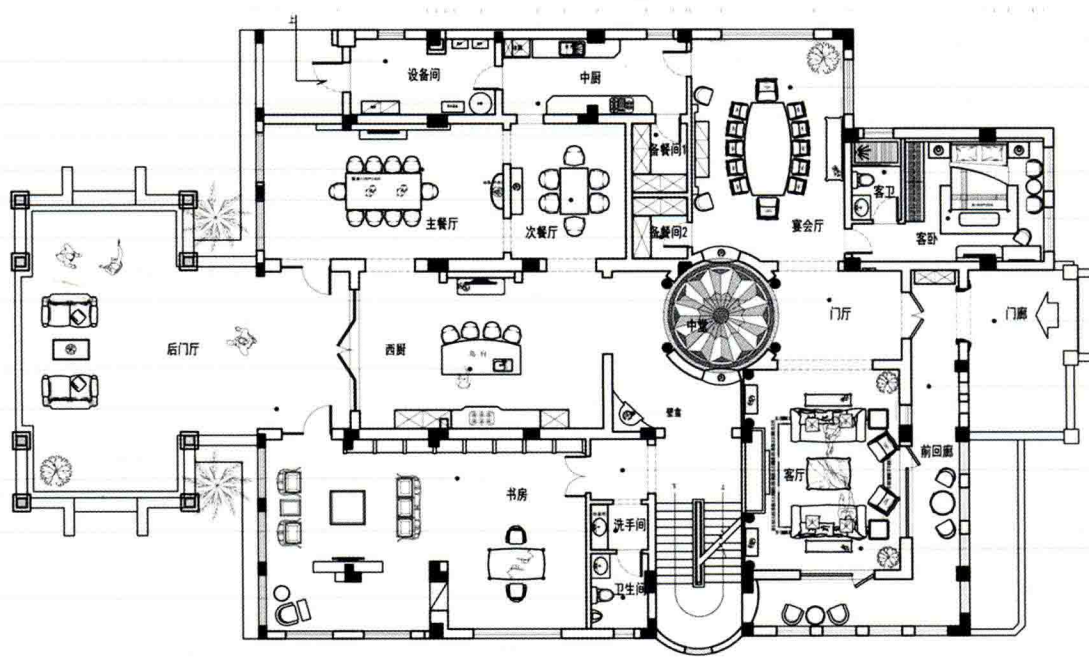
一层平面布置图
