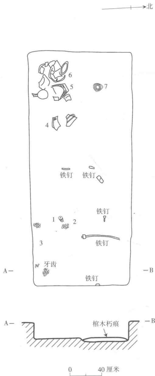
图三 M3 平剖面图
