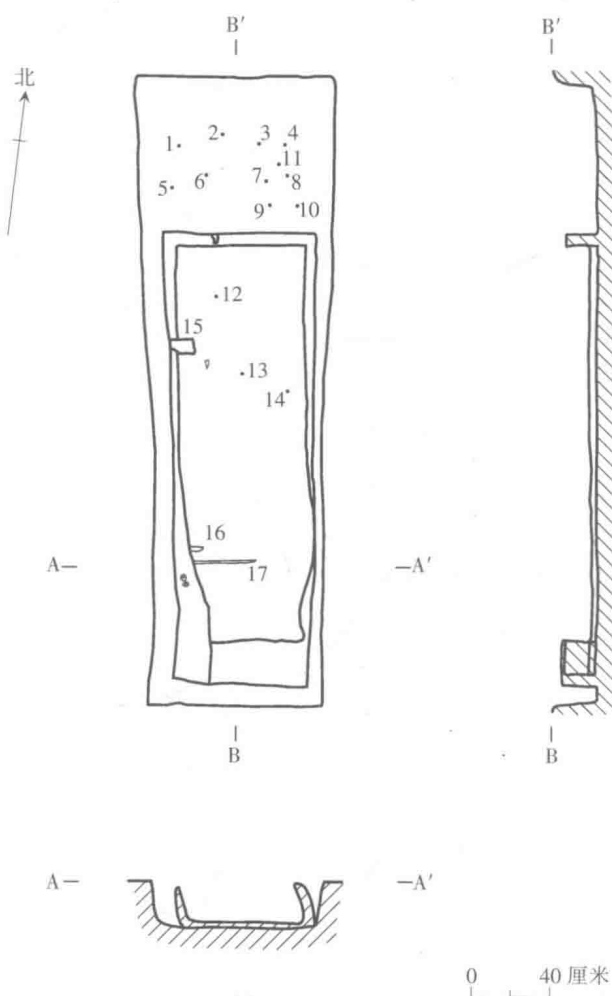
图六 M10 剖面图
