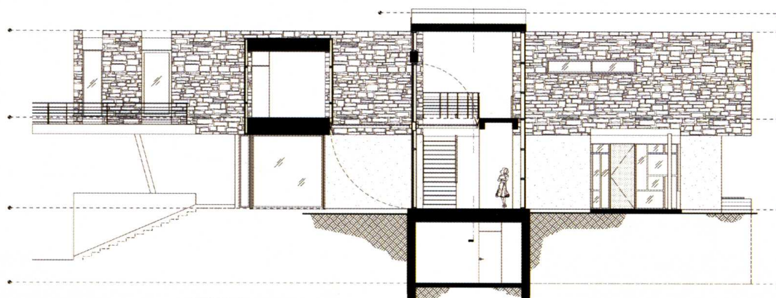
剖面图 2
