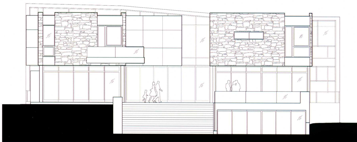
西立面图
