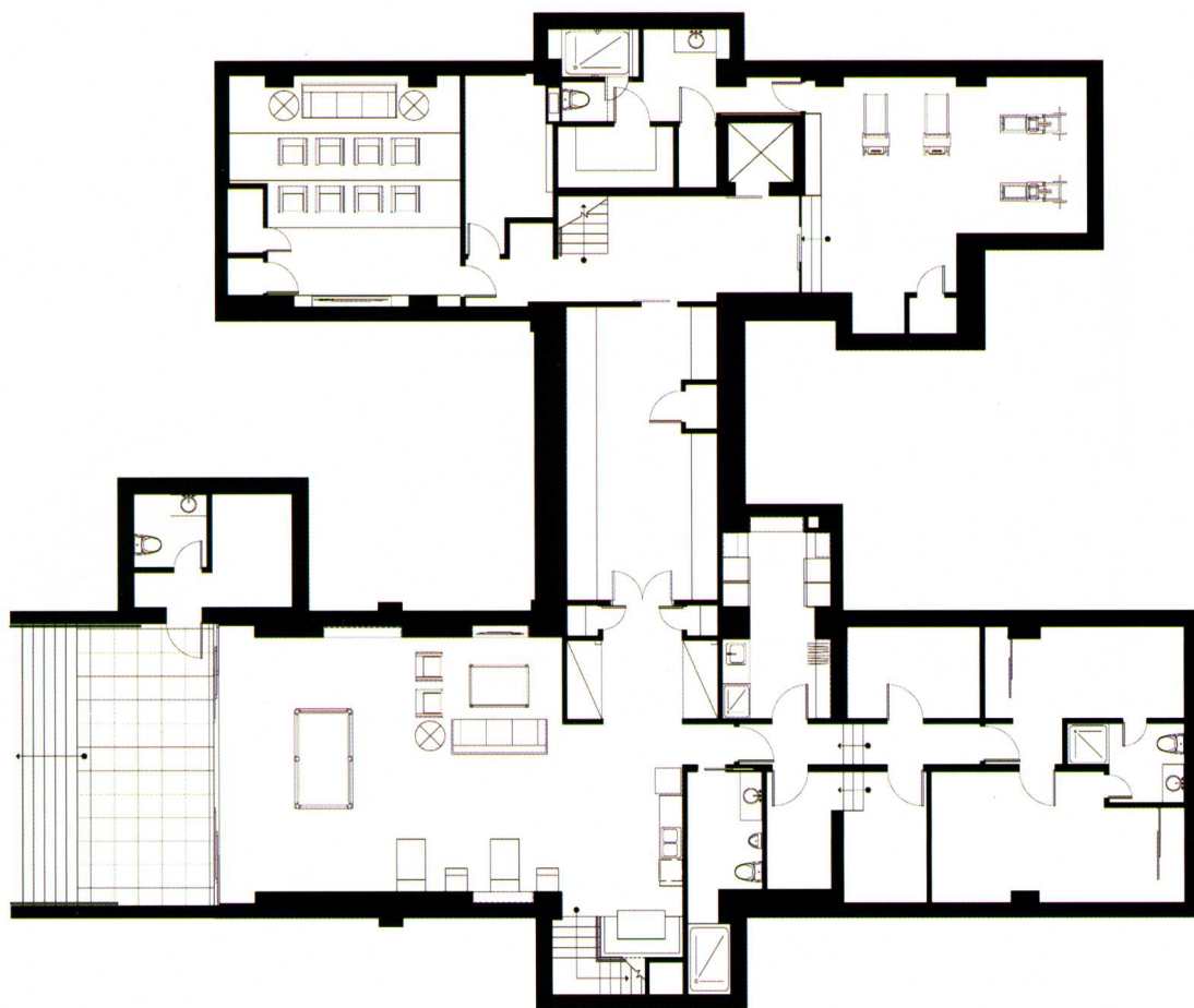
一层平面图
