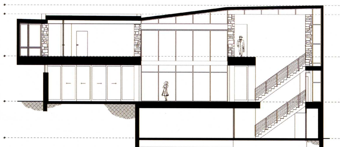
剖面图 1
