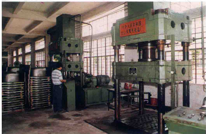
↑ 台山凤凰机电总厂自行制造的双动薄板拉伸液压机正在生产
